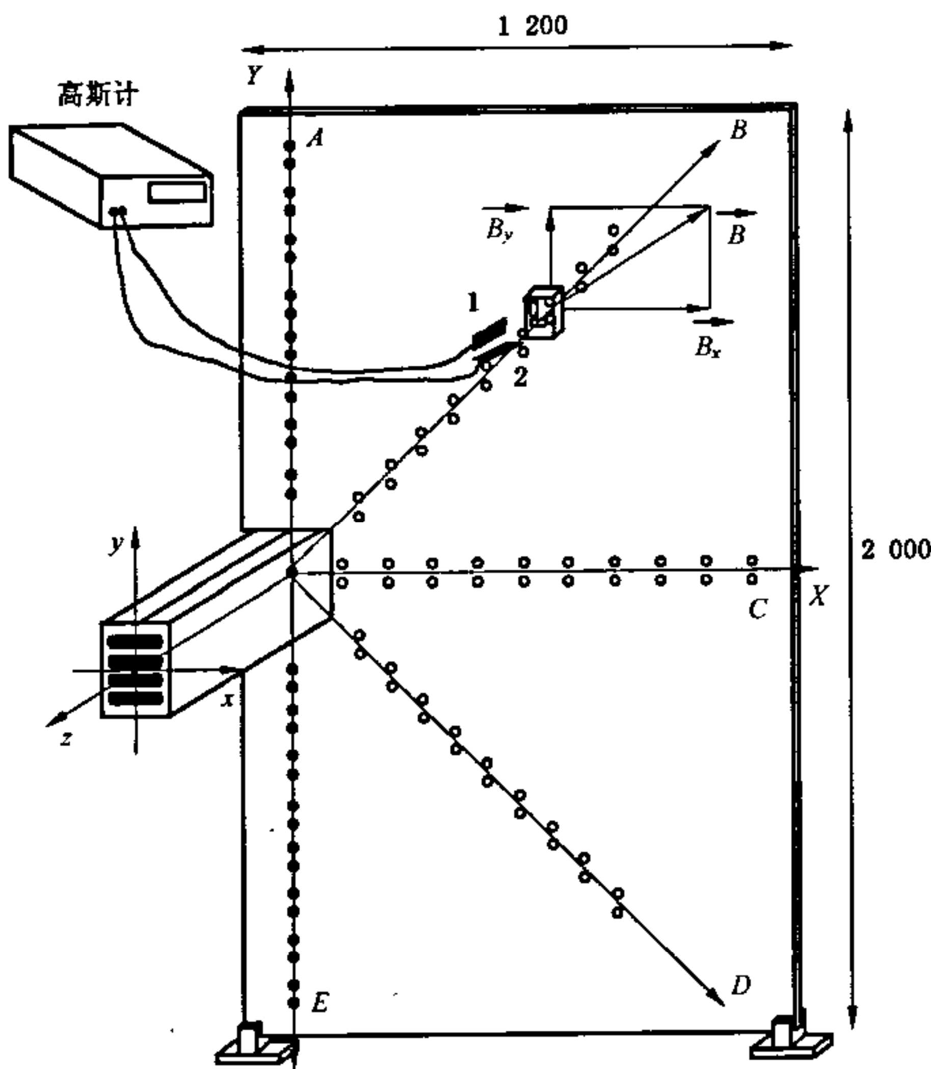
图 K.1 试验排列
