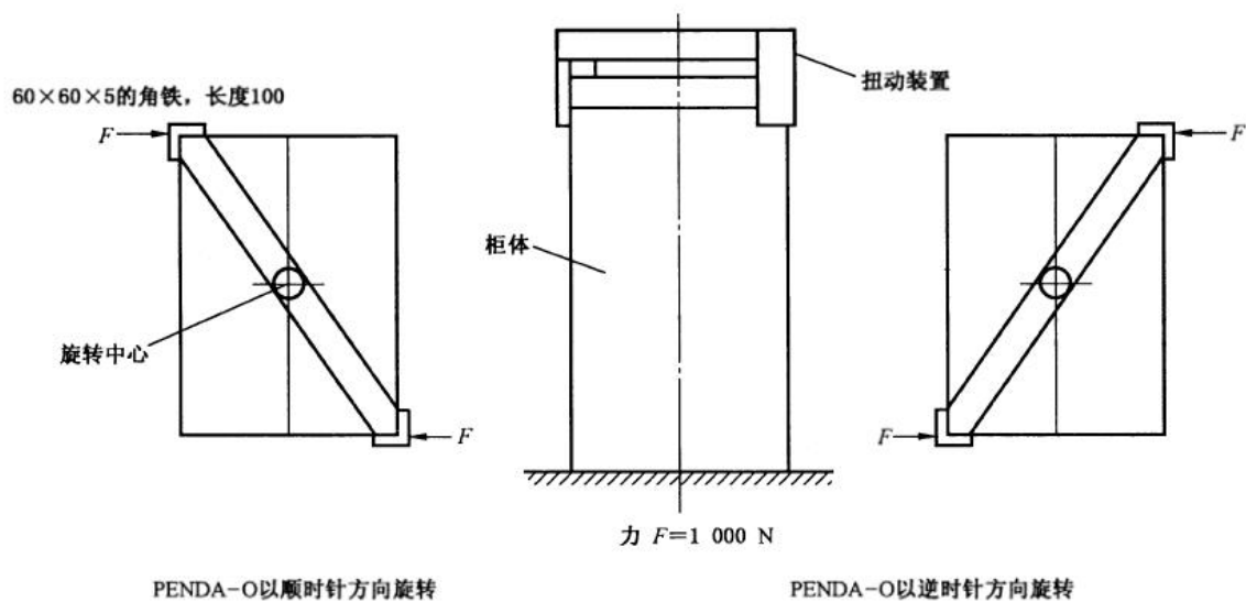
b) 不带嵌入式基座的地面安装的 PENDA-O 的耐扭力验证试验图
