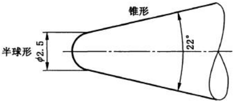
图 108 耐角状物机械撞击试验的撞击物
