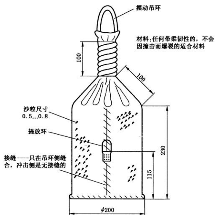
图 105 耐冲击负载验证试验的沙包图例
