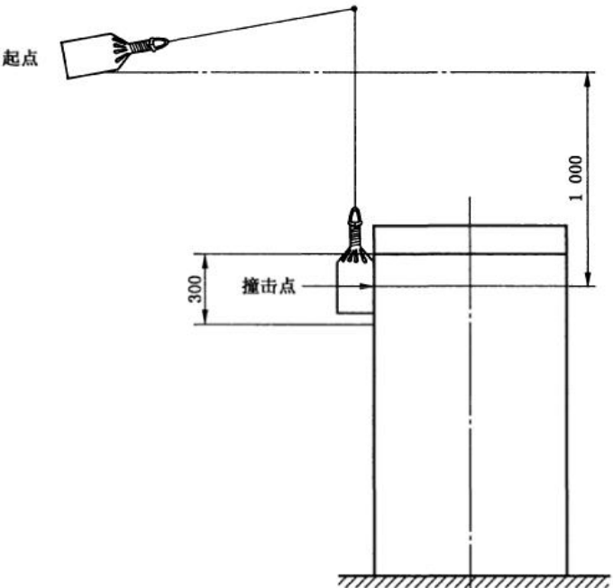
b) 不带嵌入式底座的地面安装的 PENDA-O 的耐冲击负载验证试验图
