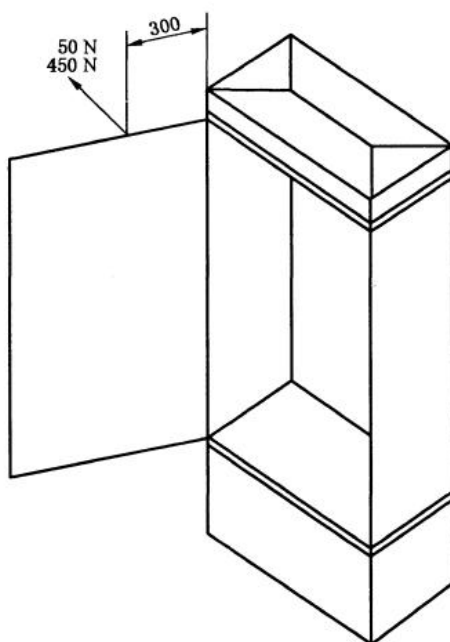
图 107 门的机械强度验证试验图
