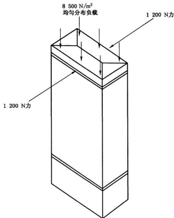
图 104 耐静负载验证试验图
