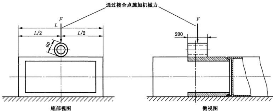
图 109 基座机械强度布置的典型试验
