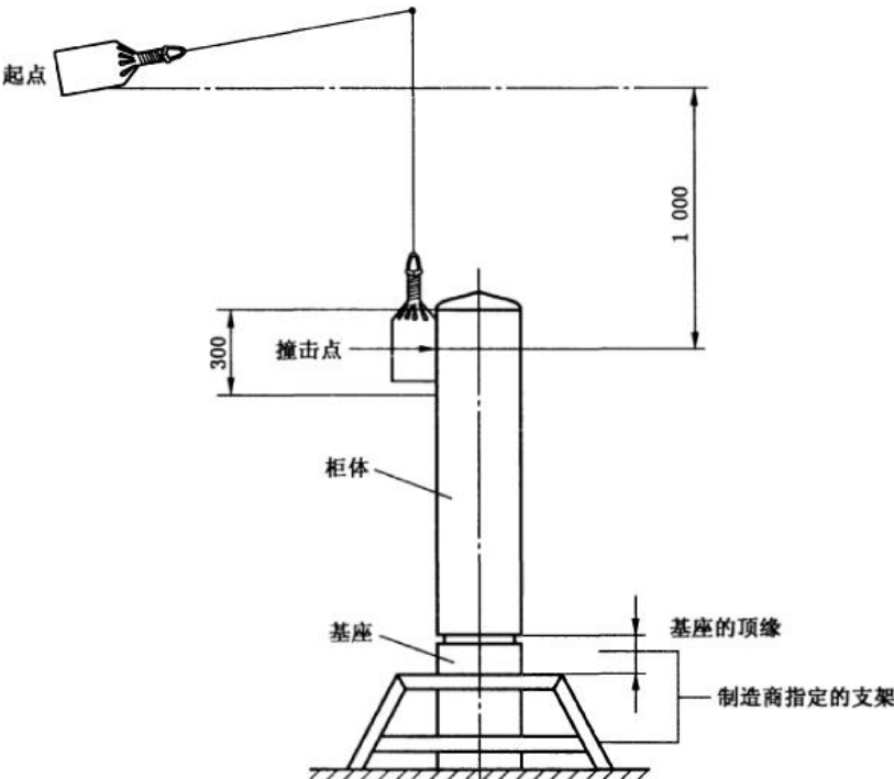
a) 带嵌入式底座的地面安装的 PENDA-O 的耐冲击负载验证试验图
